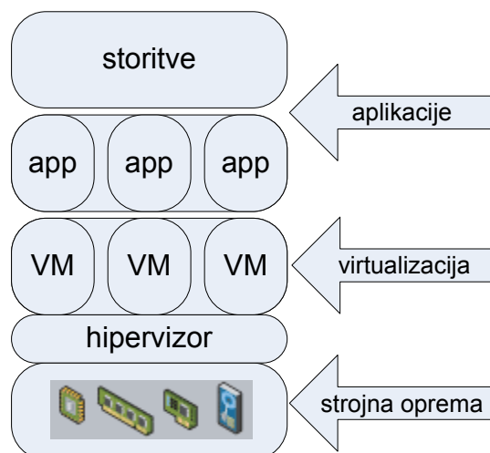
Slika 1: Koncept virtualizacije
